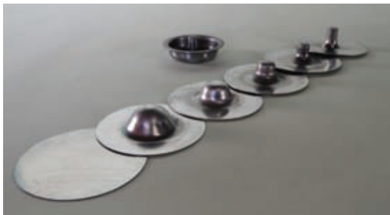
ブリキ \phi 62 \times 22h 絞りプレス 4工程 仕上げヘラ絞り 2工程
