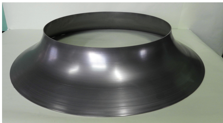
SUS304 t3.0 φ 770× 130H ヘラ絞り加工
