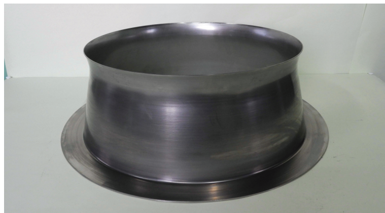
SUS304 t2.5 φ 560× 180H ヘラ絞り加工 プレス加工
